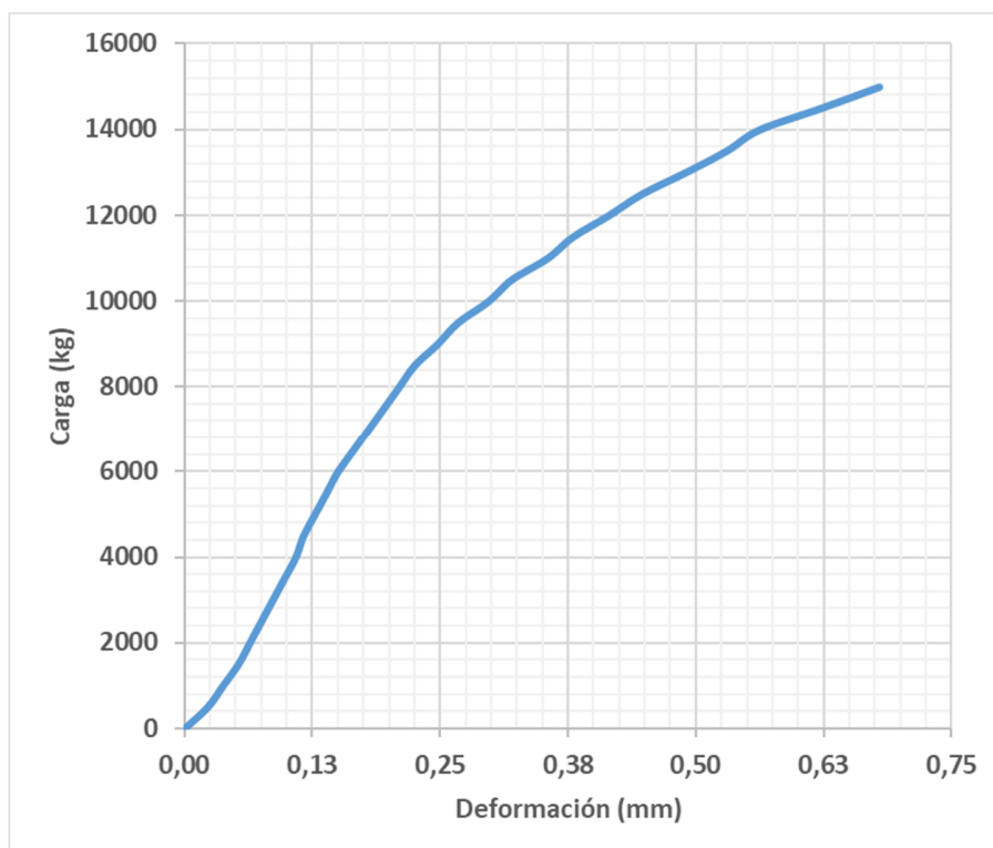
Figura 5 – Gráfico de carga-deformación en probeta 8
