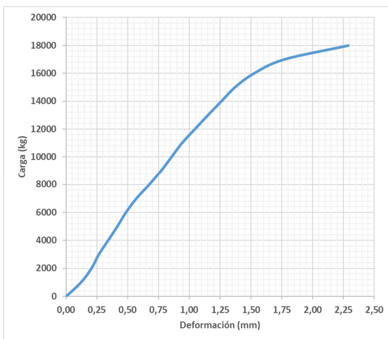
Figura 4 – Gráfico de carga-deformación en probeta 7
