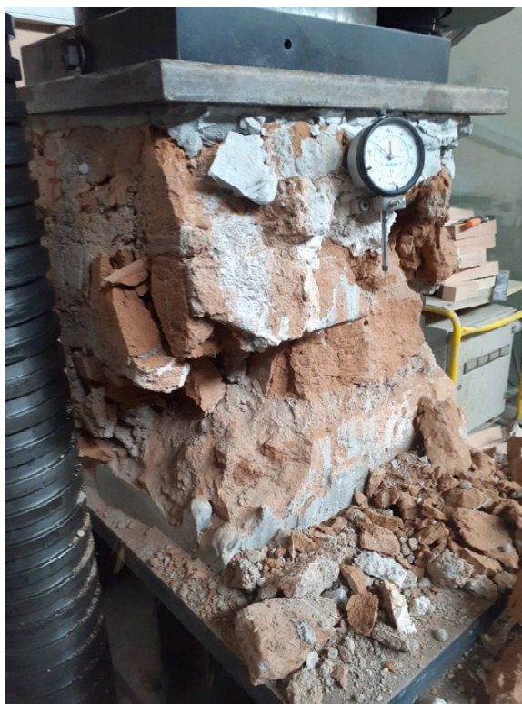
Figura 15 – Después de ensayo – Probeta 8
