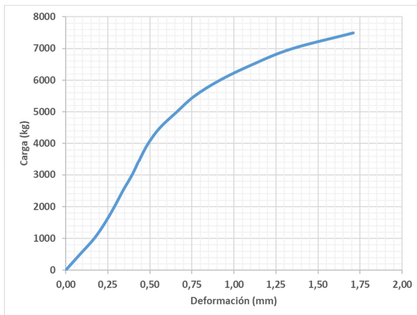
Figura 1 – Gráfico de carga-deformación en probeta 2
