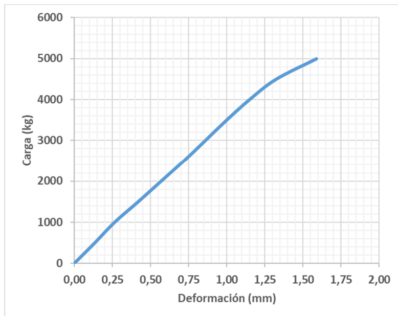
Figura 3 – Gráfico de carga-deformación en probeta 6
