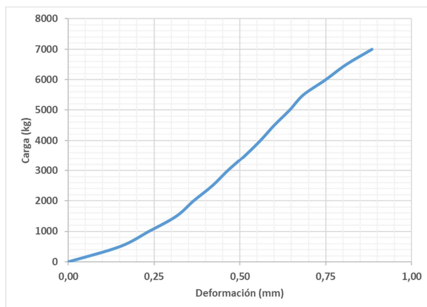
Figura 2 – Gráfico de carga-deformación en probeta 3
